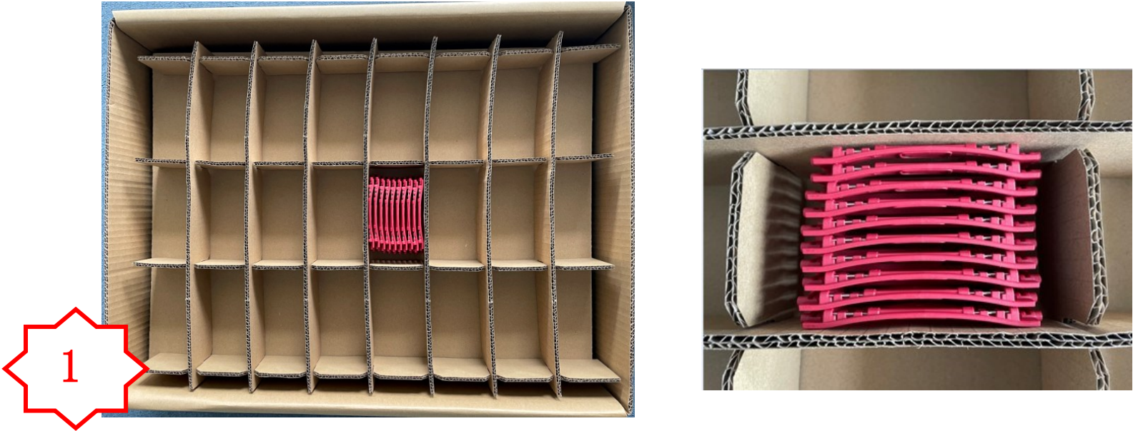
图一，每格 10 个组件，每层 24 格，每层 240pcs, 共 3 层 720pcs
